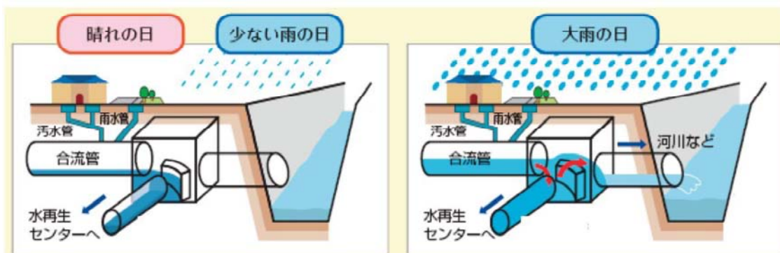
図-3.1 合流式下水道の特徴
