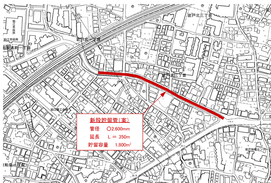
図-24 貯留管平面図
