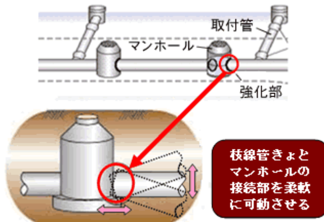
図-17.1 マンホールと管渠 きよ の接続部の可とう化イメージ 出典：国土交通省HP
