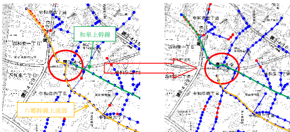
図-23.3 中和泉5丁目における対策（合流管の分水切り替え）
