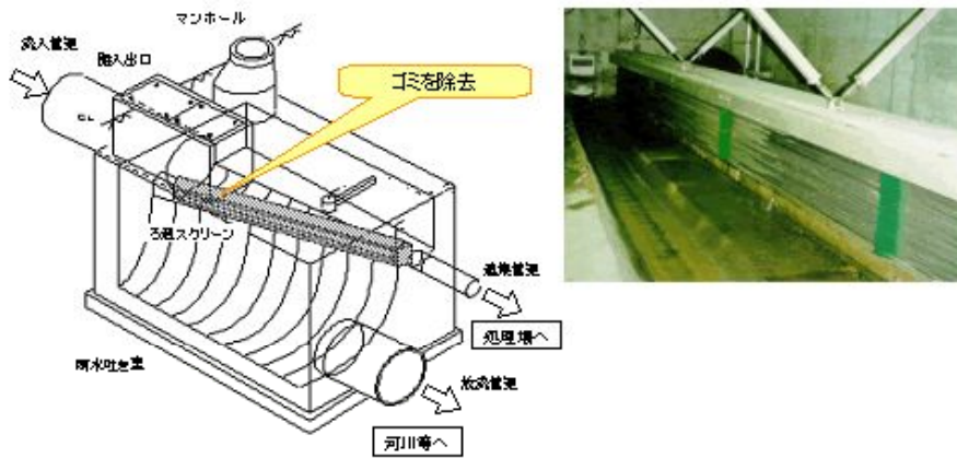
図-13.1 スクリーン施設
