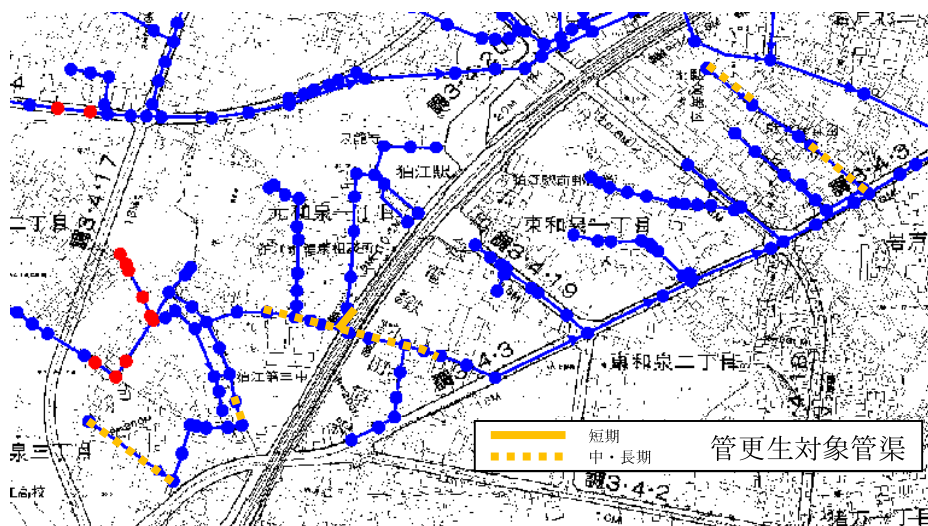
図-23.2 元和泉1丁目他における対策（管更生）
