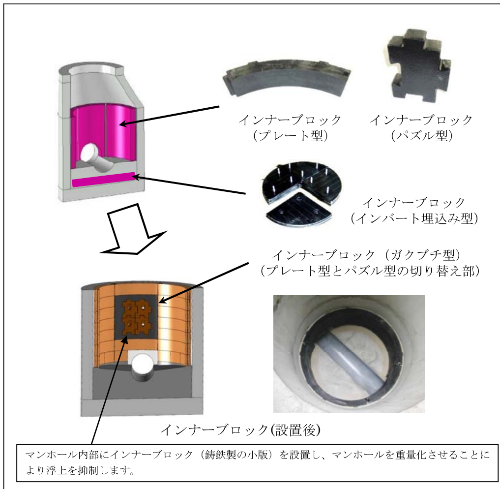
図-25 浮上防止対策工法の一例（インナーウェイト工法のしくみ）
