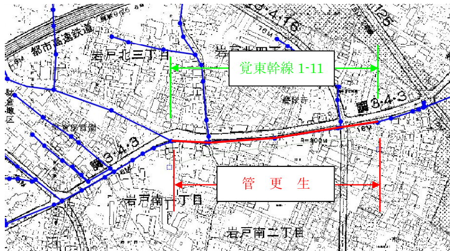
図-23.1 岩戸北4丁目における対策（管更生）
